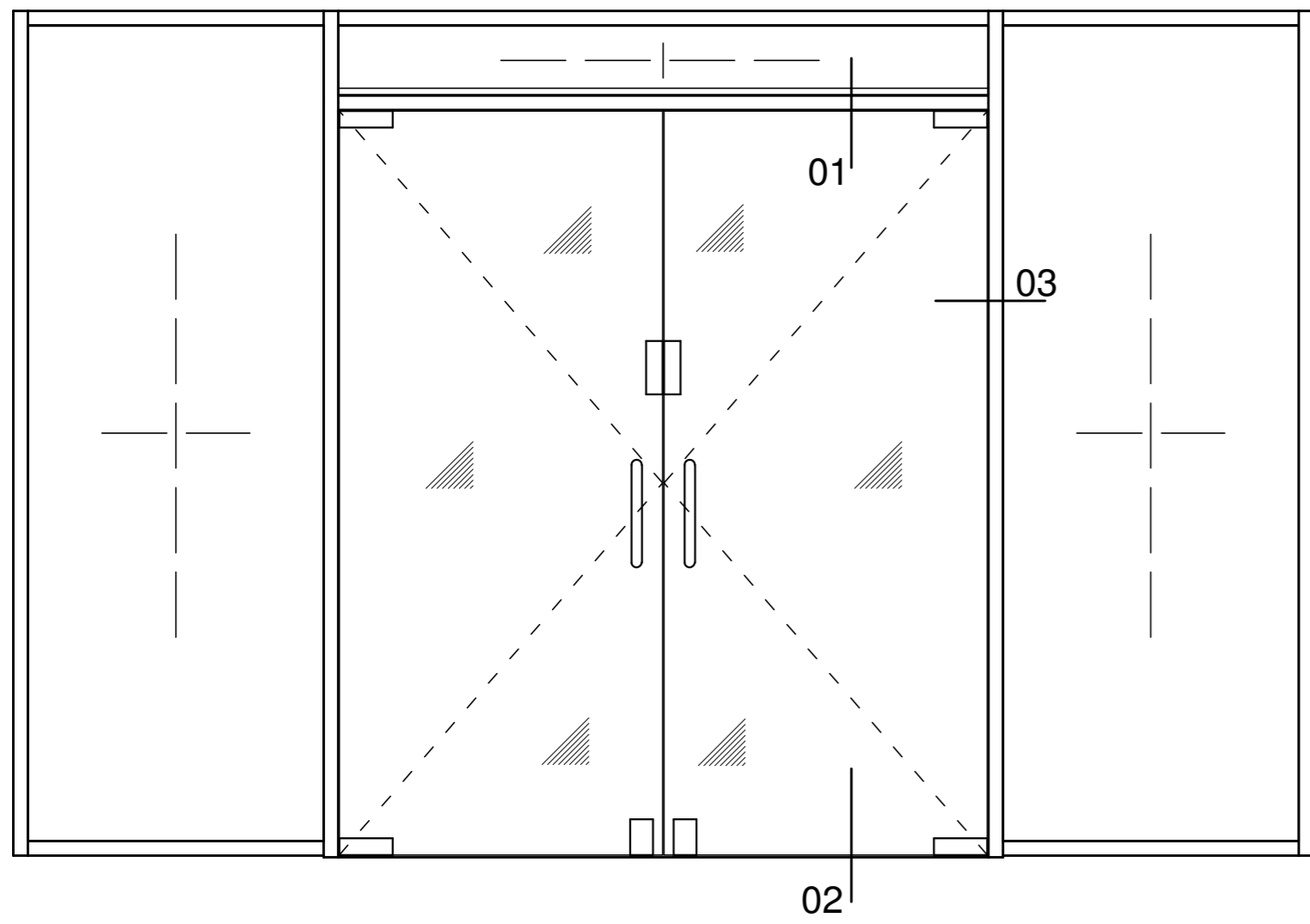
AANZICHT NL 450/VOLGLASPUI
