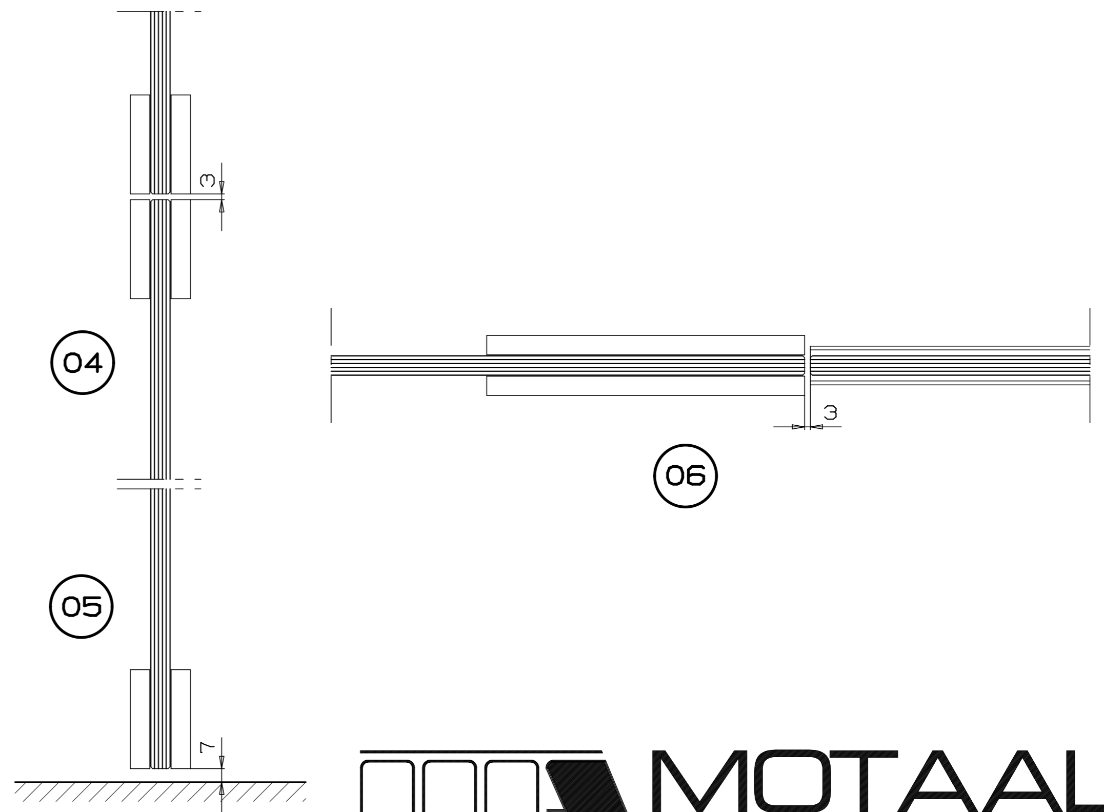
AANZICHT VOLGLASPUI
