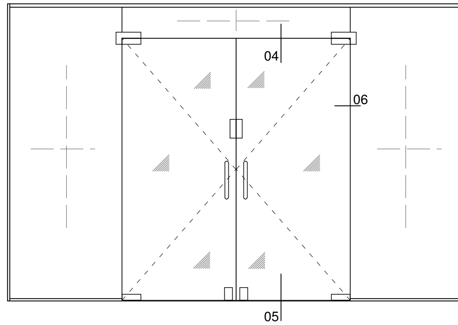
AANZICHT VOLGLASPUI
