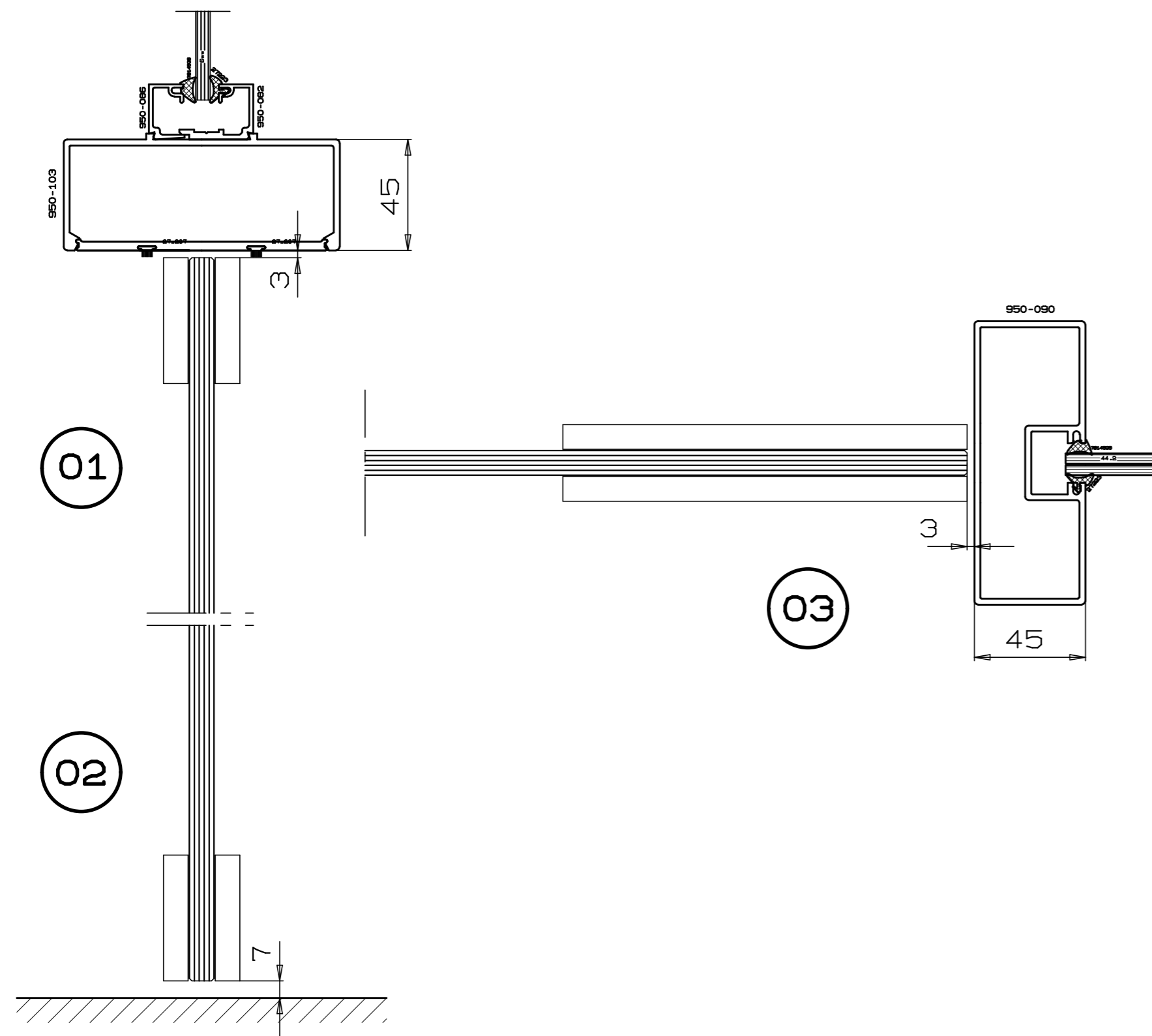
AANZICHT NL 450/VOLGLASPUI
